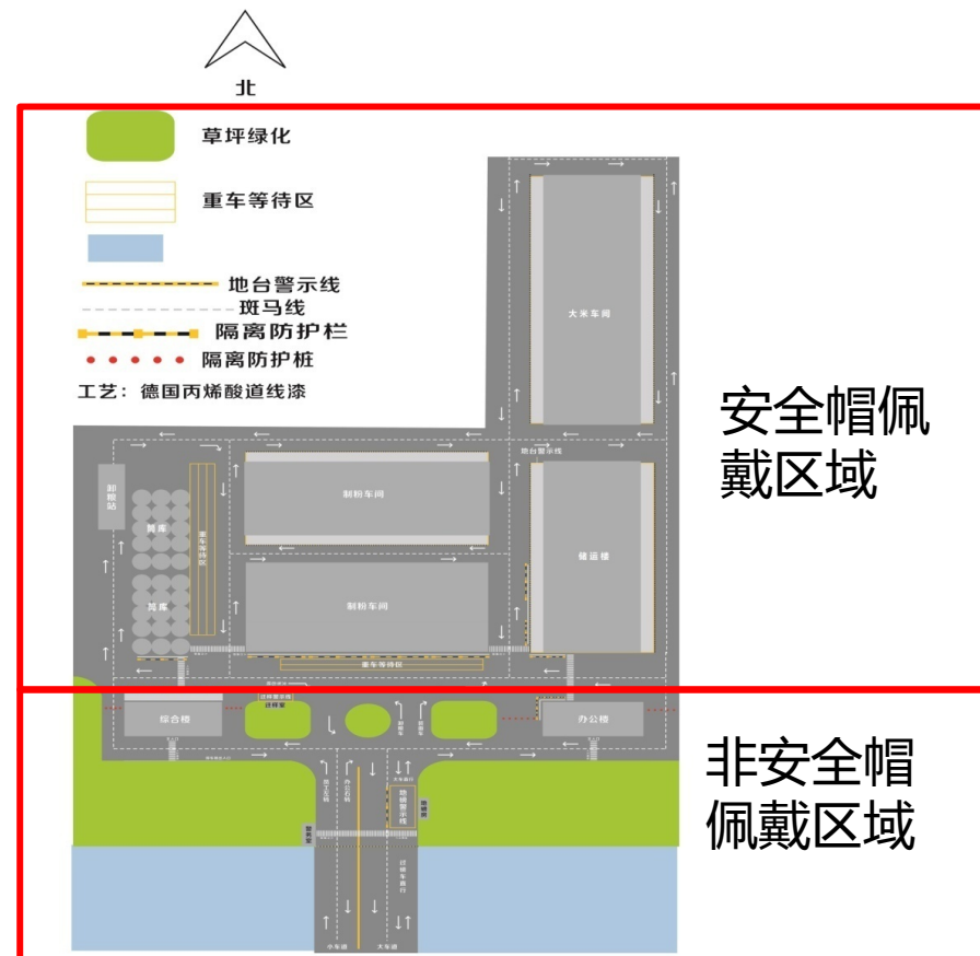
中粮利金(天津)粮油股份有限公司静海工厂道路线标系统平面分布图
